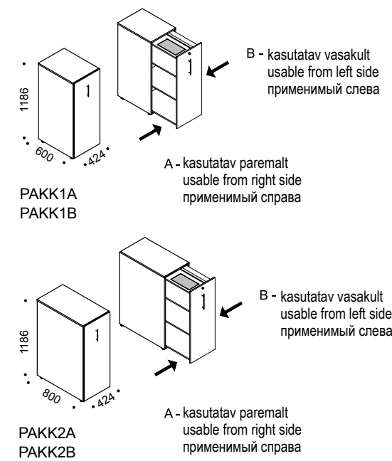
SAHTLIBOKS kappi ja konteinerisse • DRAWER UNIT for storage • ЯЩИК в шкаф и контейнер
