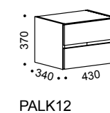
SAHTLIBOKS kappi ja konteinerisse • DRAWER UNIT for storage • ЯЩИК в шкаф и контейнер
