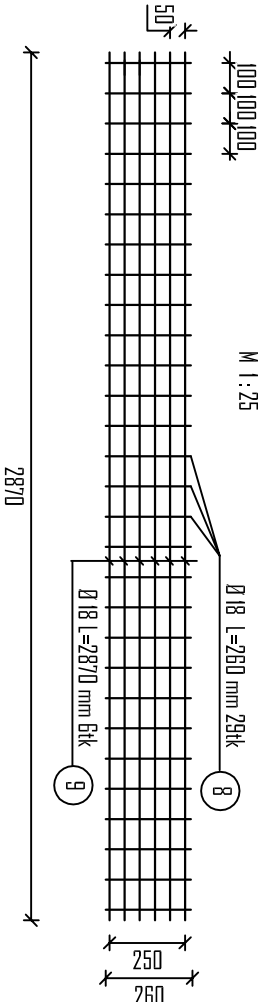
KARKASS K-3 M 1 : 25
