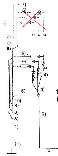
MAANDAMISE SKEEM
