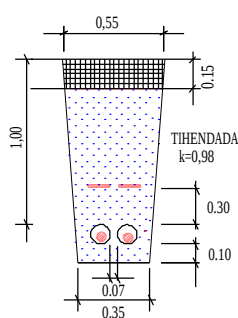
Kaks elektrikaablit kaitsetorus haljasalal
