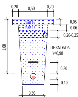
Elektri- ja sidekaabel mehaanilise kaitseta haljasalal
