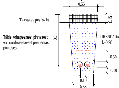
Elektri- ja sidekaabel kaitsetorus haljasalal
