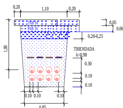
Kaheksa elektrikaablit kaitsetorus asfalsõidutee all
