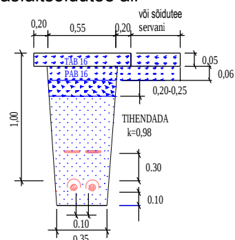
Kaks elektrikaablit kaitserennidega asfalsõidutee all
