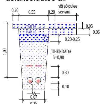
Kaks elektrikaablit kaitsetorus asfalsõidutee all
