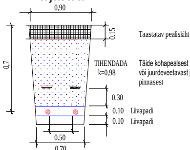
Elektri- ja sidekaabel mehaanilise kaitseta haljasalal
