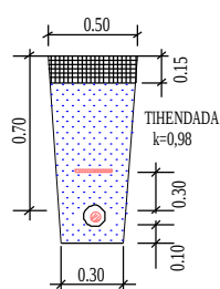
Üks elektrikaabel kaitsetorus haljasalal
