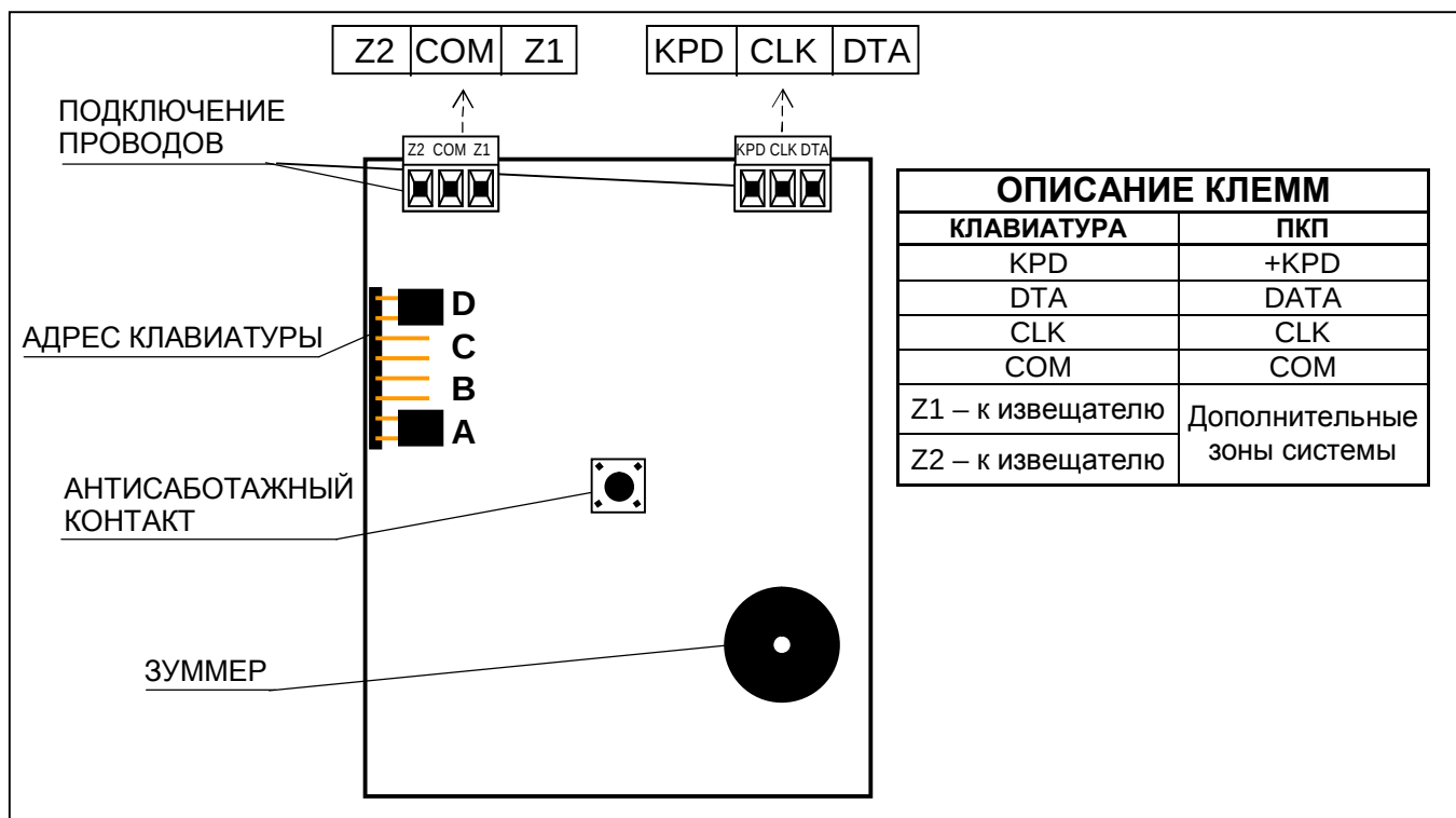
Рис. 5. Вид платы клавиатуры CA-6 KLED-S.
