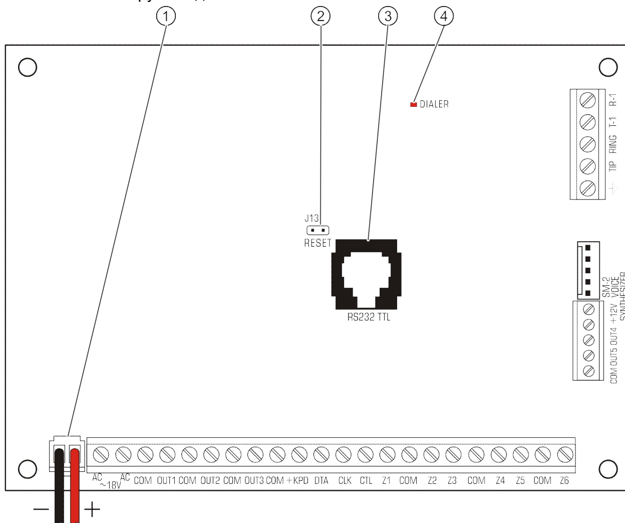
Рисунок 2. Вид платы ПКП CA-6
