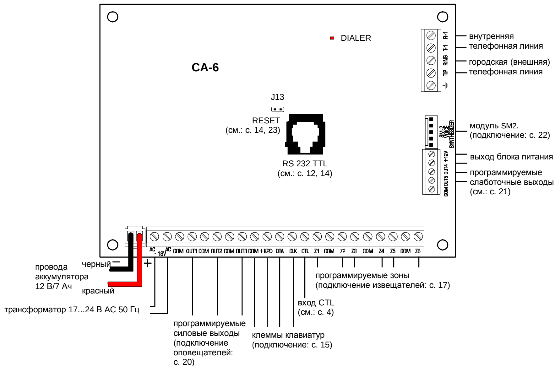
Схематичный вид приемно-контрольного прибора СА-6 (детальное описание клемм основной платы см.: с. 14).
