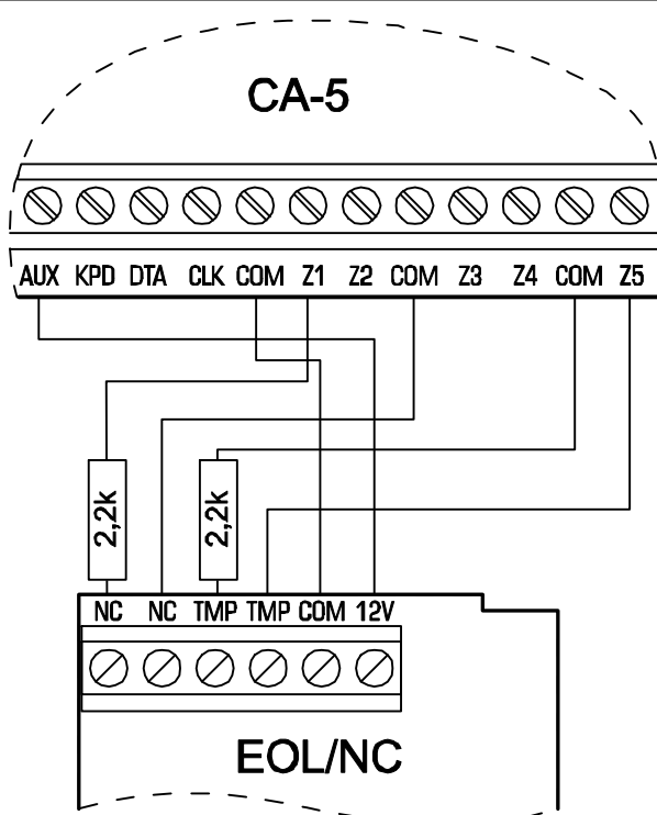
Рис. 8. Пример подключения к ПКП извещателя по схеме с оконечным резистором EOL/NC.
