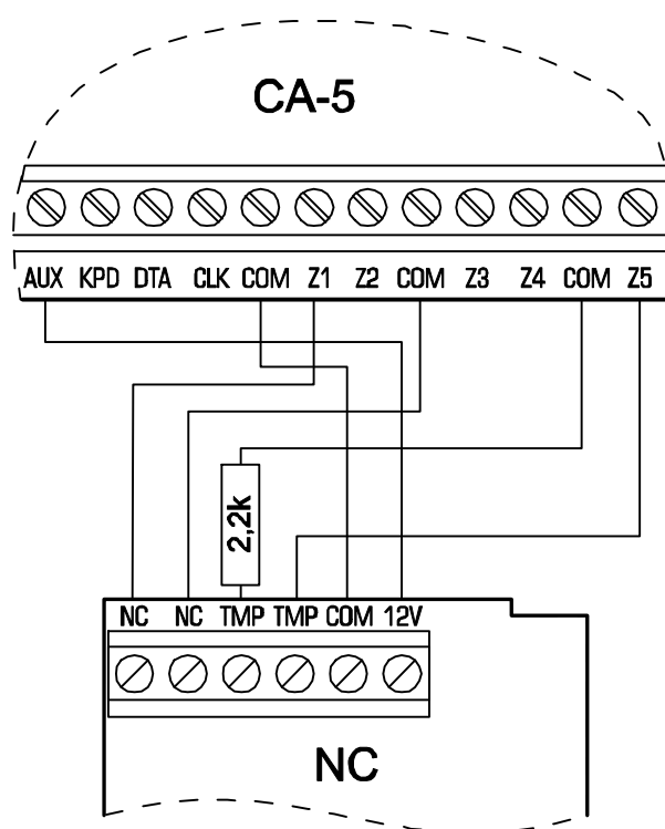
Рис. 6. Пример подключения к ПКП извещателя по схеме NC (извещатель NO подключается идентично).
