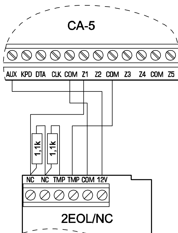
Рис. 9. Пример подключения к ПКП извещателя по схеме с двумя оконечными резисторами 2EOL/NC (извещатель NO подключается идентично).
