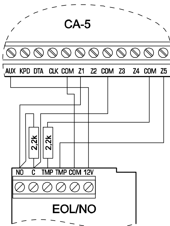
Рис. 7. Пример подключения к ПКП извещателя по схеме с оконечным резистором EOL/NO.
