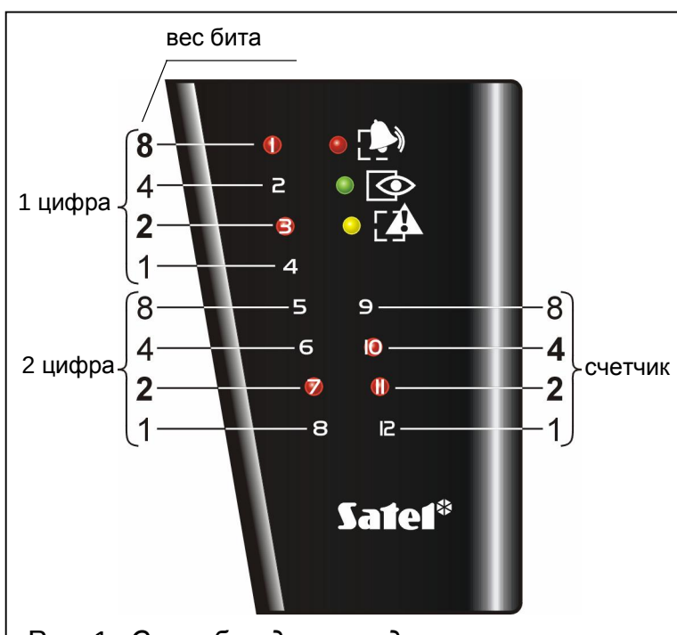
Рис. 1. Способ индикации данных на примере клавиатуры CA-10 KLED. Программируется шестой параметр (счетчик = 6), светодиоды 1-8 показывают текущее значение параметра = A2 (HEX)
