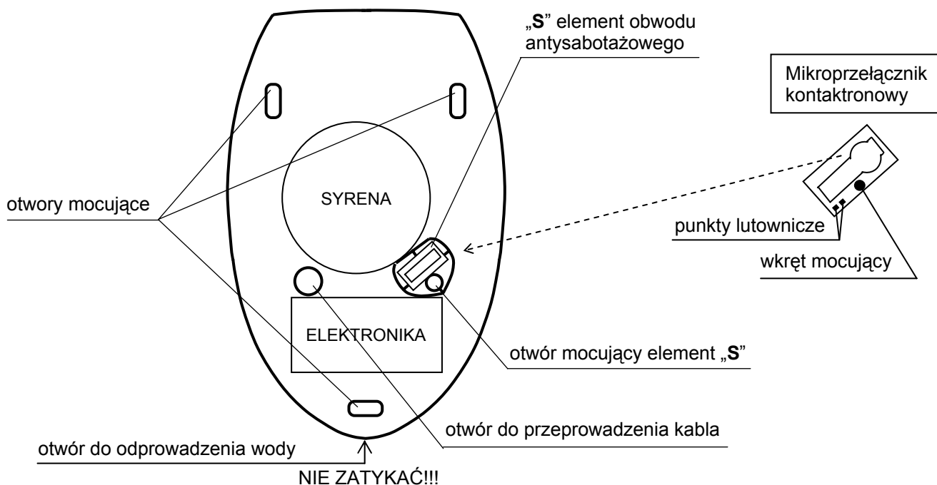
Rysunek 1. Widok podstawy obudowy sygnalizatora
