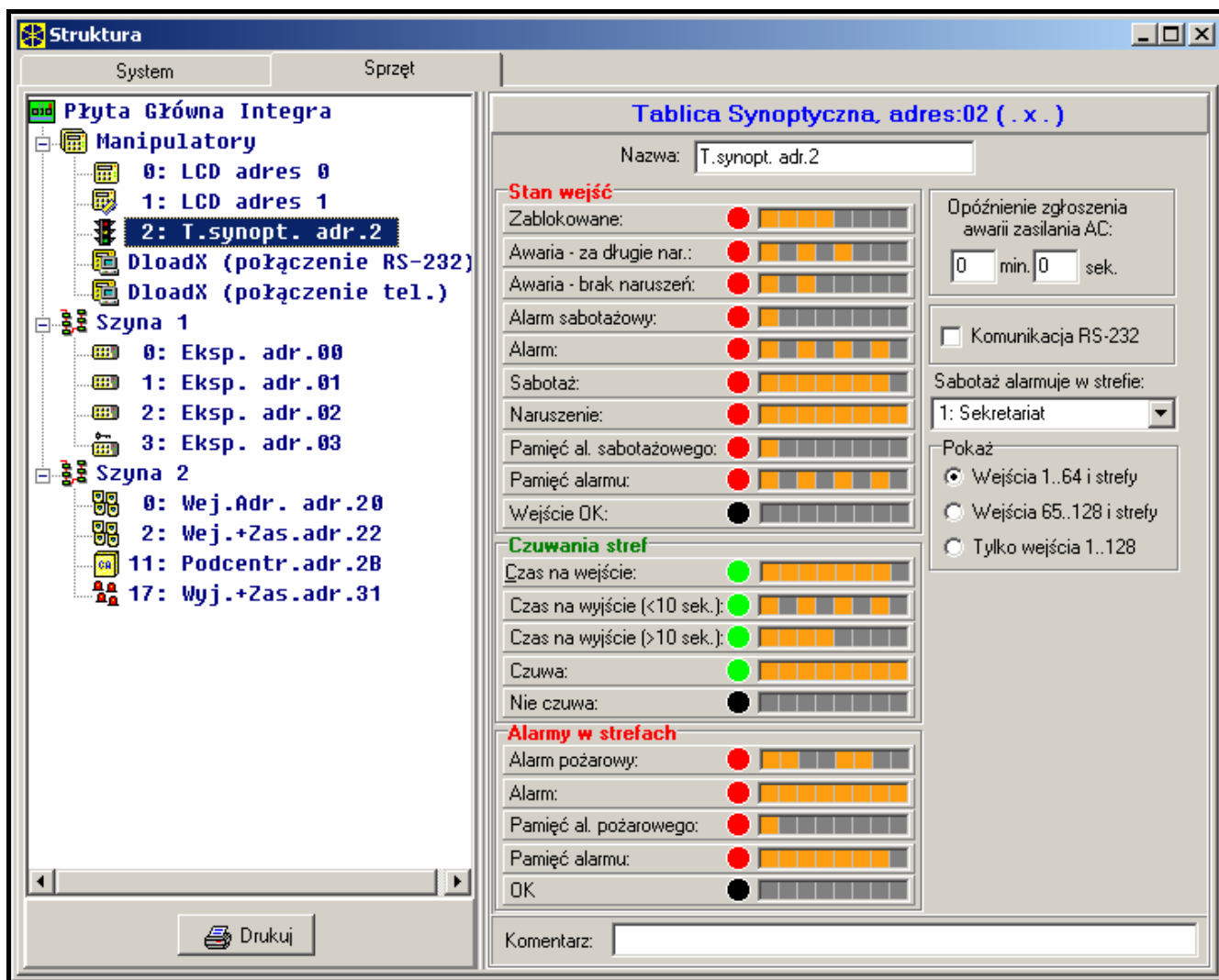
Rysunek 4. Programowanie ustawień tablicy synoptycznej w programie DloadX dla centrali INTEGRA 128.
