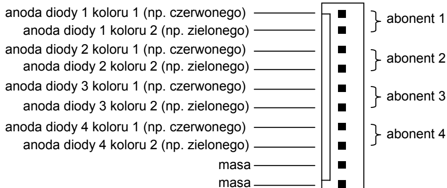
Rysunek 6. Sposób podłączenia diod LED do styków gniazda J1 tablicy synoptycznej w przypadku współpracy ze stacją monitorującą STAM-1.
