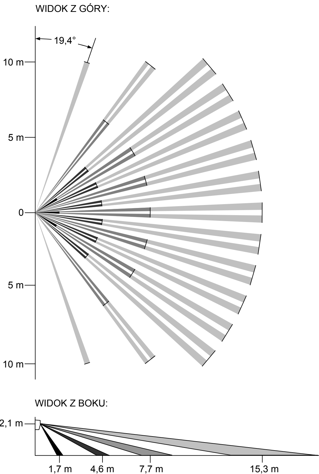
Rys. 3. Rozkład wiązek i zasięg czujki z soczewką typu ekstra szerokokątna (EWA).
