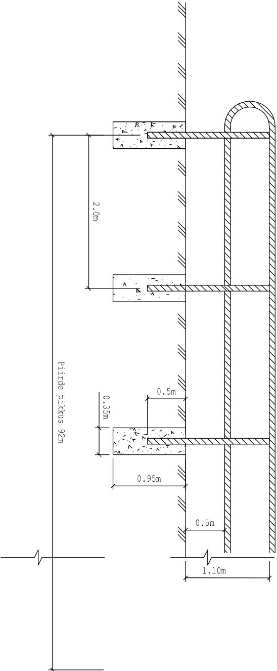
EXAMPLE OF ZINC COVERED TUBULAR FENCE, Ø 76mm/ TSINGITUD TORUPIIRDE NÄIDIS, Ø 76mm M 1:50
