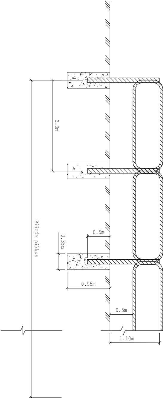
EXAMPLE OF ZINC COVERED TUBULAR FENCE, Ø 60mm/ TSINGITUD TORUPIIRDE NÄIDIS, Ø 60mm M 1:50
